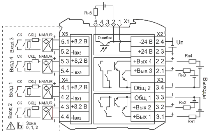
Рисунок 6.4 – Типовые схемы подключения барьеров KA5234Ex-NN
