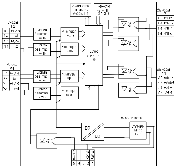
Рисунок 5.3 – Функциональная схема барьера КА5234Ех-12
