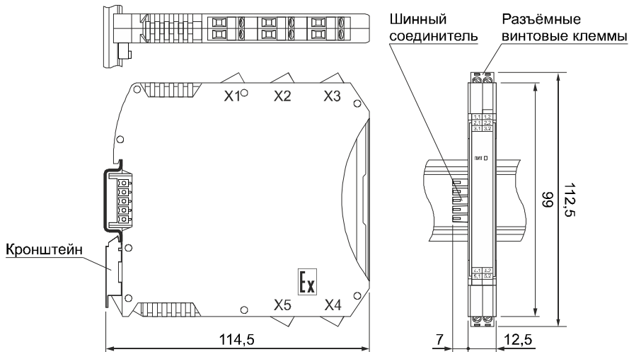
Рисунок 6.1 – Габаритные размеры барьера KA5232Ex-NN
