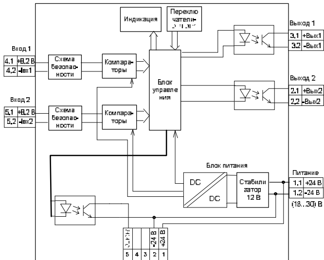
Рисунок 5.2 – Функциональная схема барьера KA5232Ex-12
