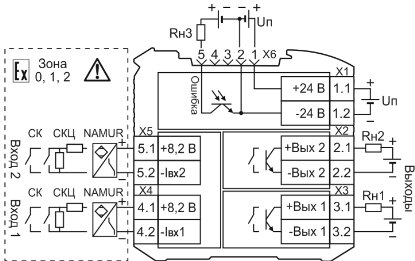
Рисунок 6.3 – Типовые схемы подключения барьеров KA5232Ex-NN
