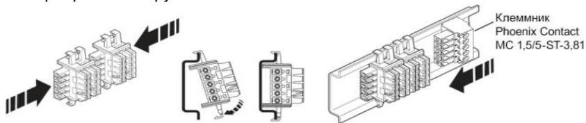
Рисунок 6.5 – Установка шинных соединителей на DIN- рейку
